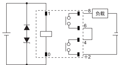
图2.反极性
