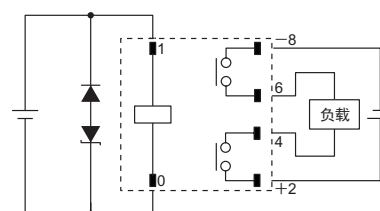
图4.反极性
