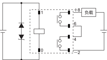
图1.正极性
