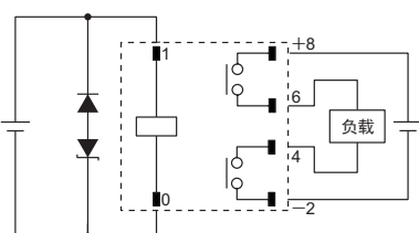
图3.正极性
